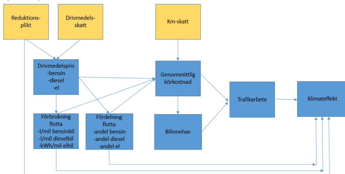
Figur 6. Schematisk uppbyggnad av scenarioverktyget för effektbedömning av styrmedelspaket
